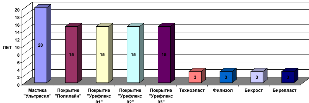
Срок службы кровельных материалов до ремонта, лет
