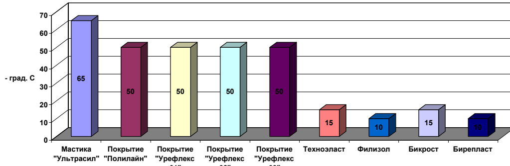
Морозостойкость -С кровельных материалов
